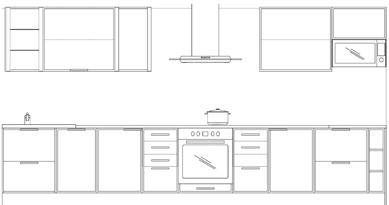
Общая длина кухонного гарнитура 4232 мм. Вариант 5.
