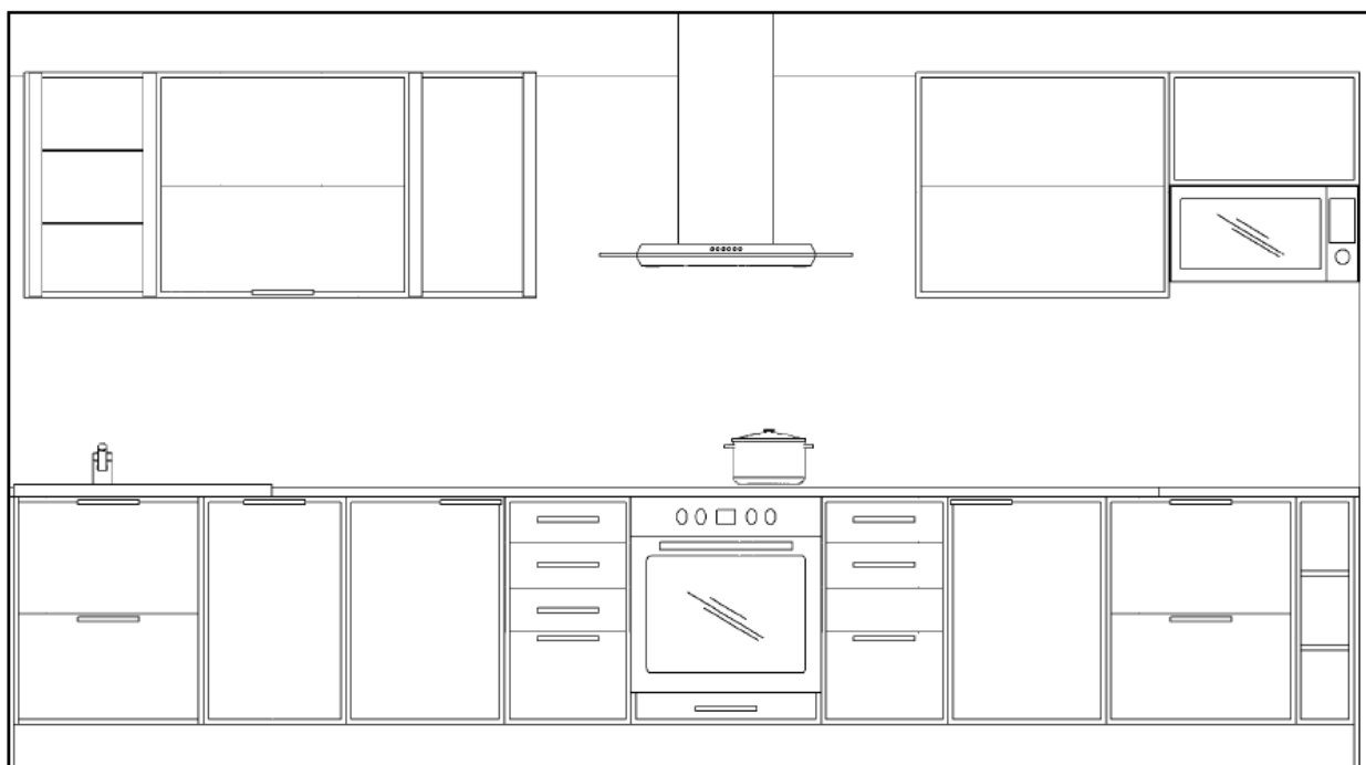
Общая длина кухонного гарнитура 4232 мм. Вариант 5.
